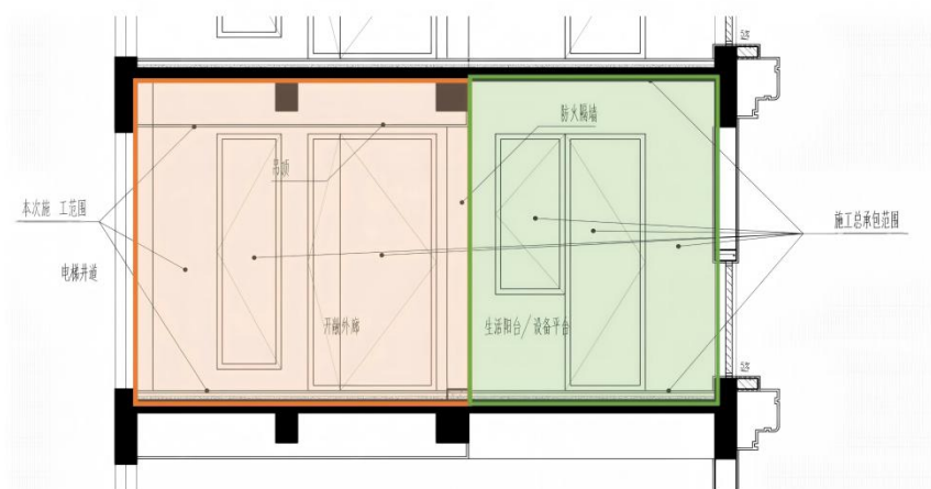
1-1剖面示意
