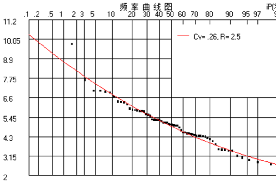
图 错误!文档中没有指定样式的文字。-1 开垦河年径流量 P—Ⅲ型曲线图
