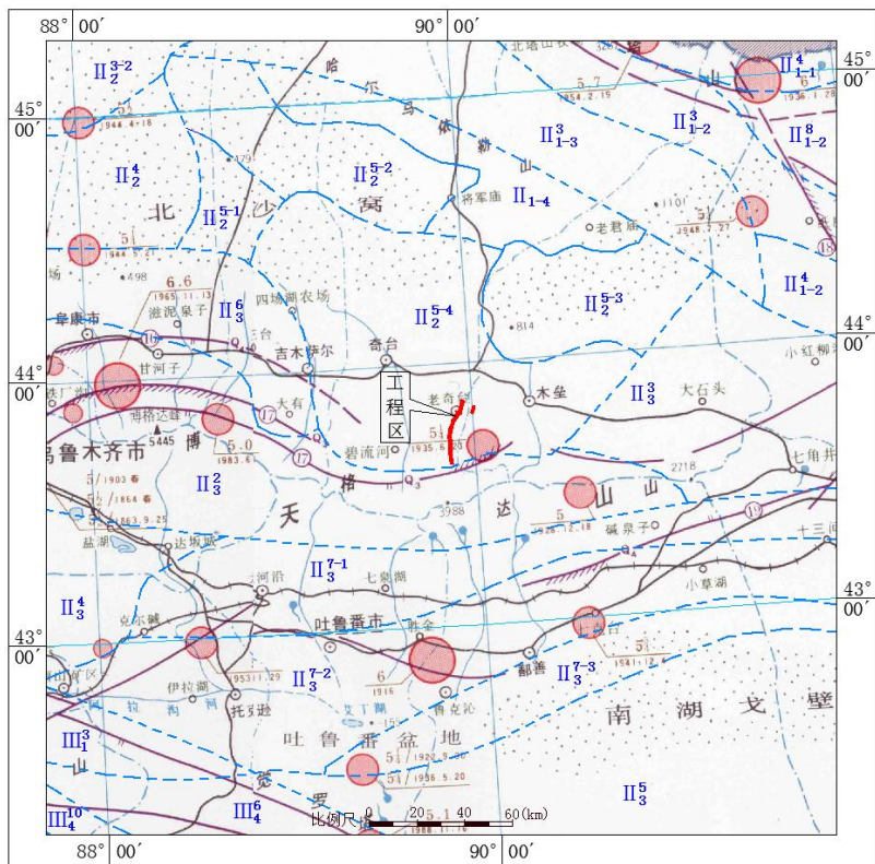
图 错误!文档中没有指定样式的文字。-2 区域构造与地震震中分布图
