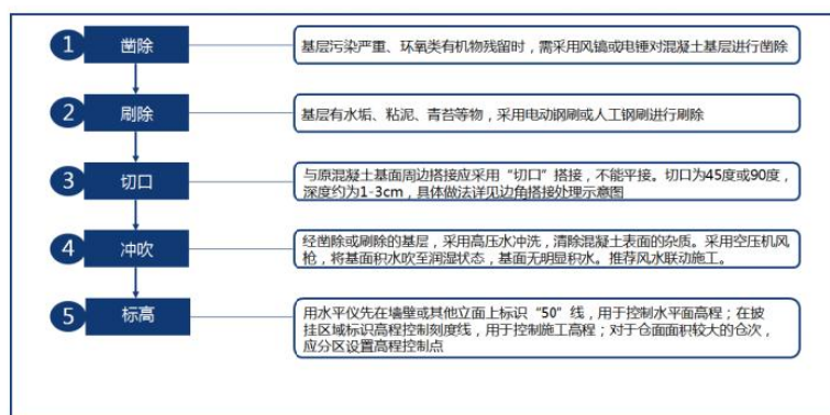
图 2.2.2-2 仓面准备工序
