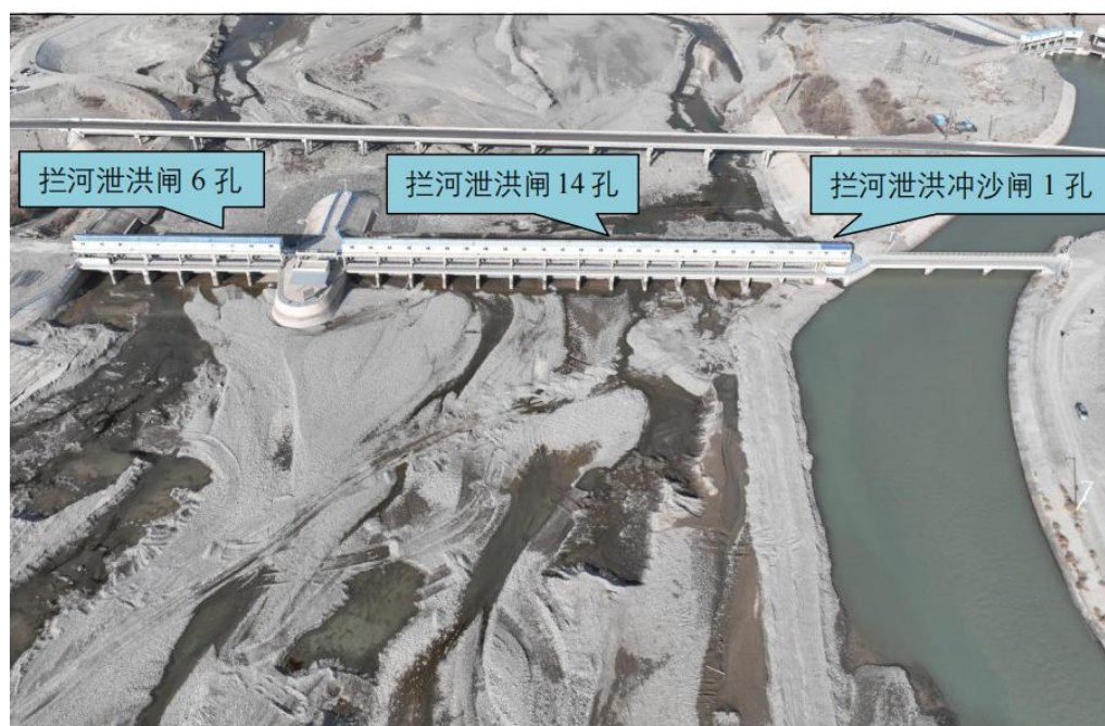
图 1-2 秋格尔引水枢纽工程现状
