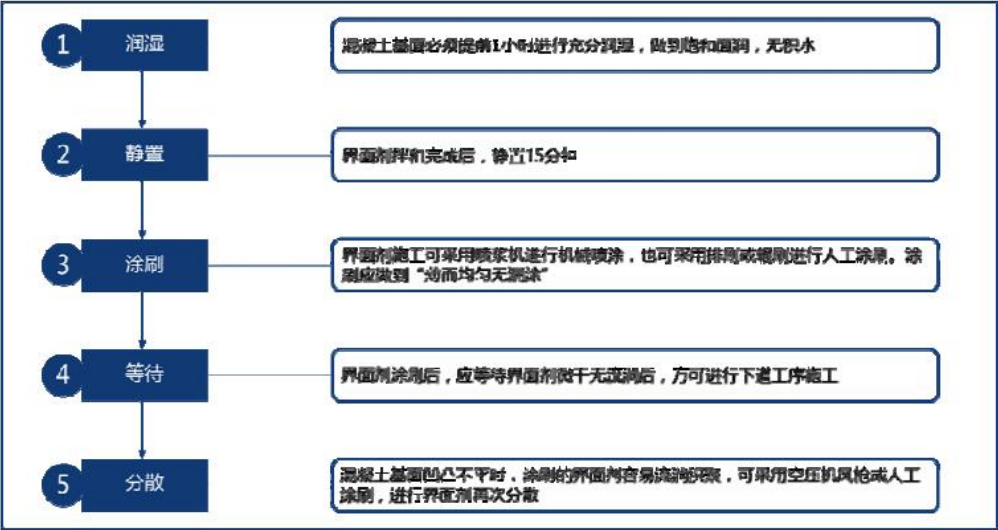
图 2.2.1-4 界面处理工序
